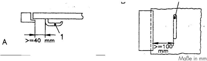
Bild 19: Positionierung von Griffen
