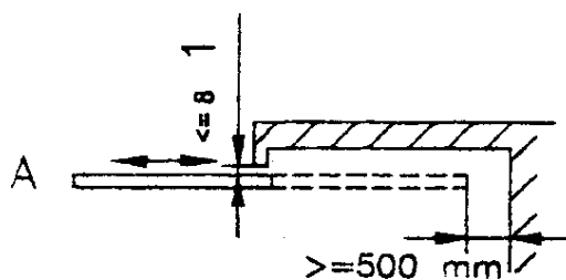
Bild 17: Einzugsstellen zwischen Flügel und Wand
