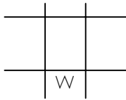
Bild 13: Sicherheitsabstände an rechteckigen Durchgriffsöffnungen
