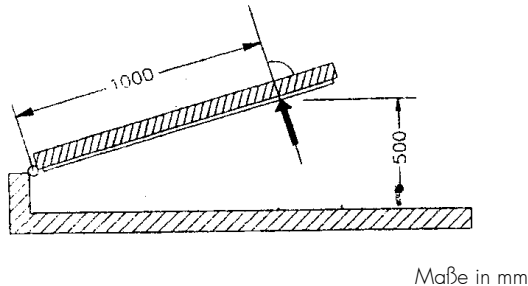
Bild 15: Kraftbegrenzung zwischen Flügel und Umgebung
