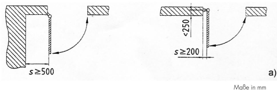
Bild 14: Sicherheitsabstände an Drehflügeltoren (im Bild Buchstabe a) streichen)
